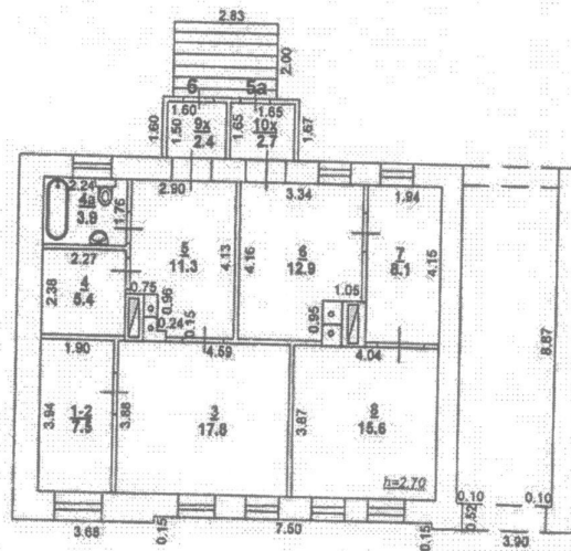
Литера А 1 этаж
