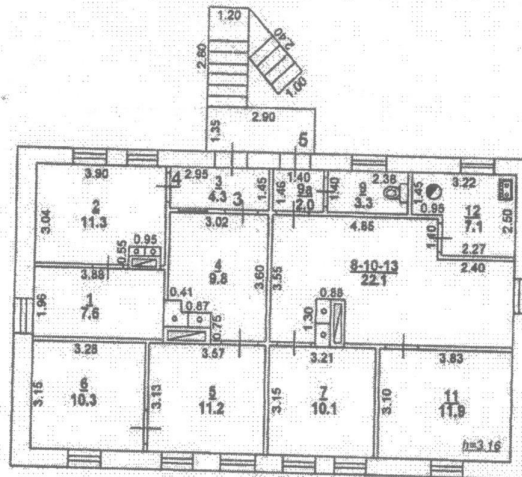
Литера А 2 этаж
